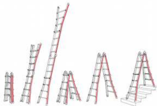
Strichzeichnung der Verwendungsmöglichkeiten der Teleskopleiter „Telestep®“ 4042 von Hymer-Leichtmetallbau
